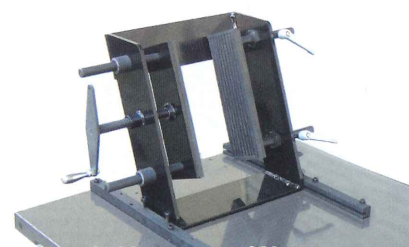
前輪クランプ装置 ※オプション品
